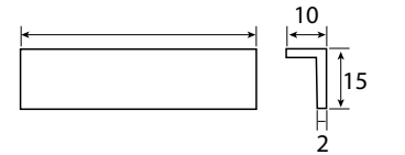
Borde ingletado (H=5) Step squared edge
