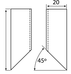
Borde ángulo interior ingletado Step angle interior squared edge
